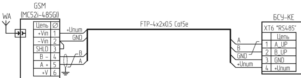
Рисунок Г.2 – Схема подключения GSM-извещателя MC52i-485GI.
