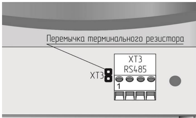
б) пульт
