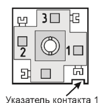
Розетка G2U3000-SK-1G
