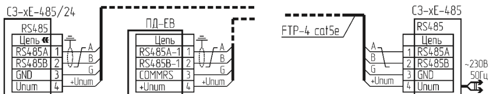
Рисунок В.3 – Нумерация контактов разъемов. Вид со стороны пайки (монтаж).
