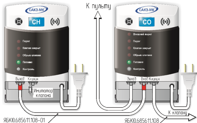
Рисунок Б.1 – Типовая схема соединений
