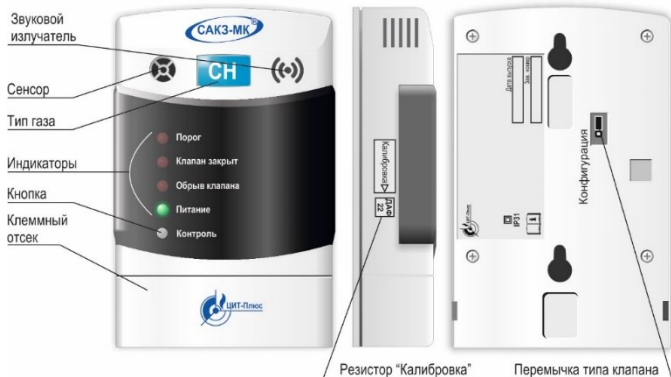
Рисунок 1 – Внешний вид сигнализатора
