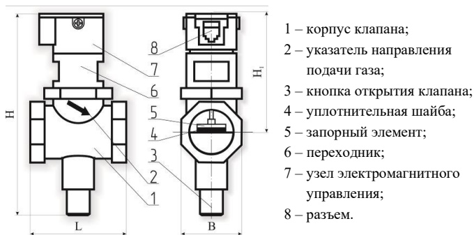
Рисунок 3 – Внешний вид клапана КЗЭУГ.
