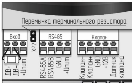
а) сигнализатор
