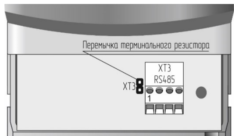
б) пульт
