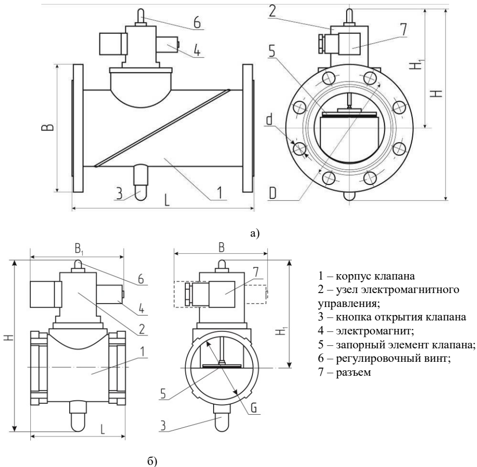
Рисунок 2 – Внешний вид клапана: а) фланцевый; б) муфтовый
