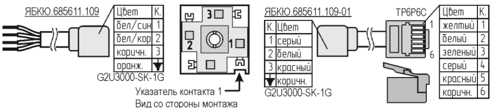
Рисунок 3 – Схема кабелей ЯБКЮ.685611.109 и ЯБКЮ.685611.109-01.
