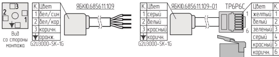
Рисунок 3 – Схема кабелей ЯБКЮ.685611.109 и ЯБКЮ.685611.109-01.
