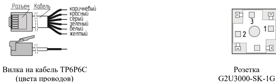
Рисунок А.3 – Нумерация разъемов кабелей.
