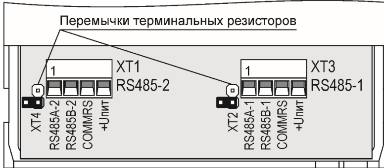
Рисунок Г.6 – Расположение разъемов в клеммном отсеке БС-01(02)
