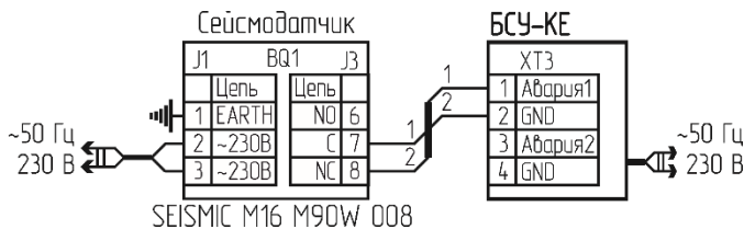
Рисунок 22 – Схема подключения сейсмического сенсора SEISMIC M16 M90W 008.
