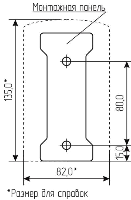
Рисунок Г.1 – Разметка отверстий для крепления сигнализаторов СЗ-хЕ, пульта
