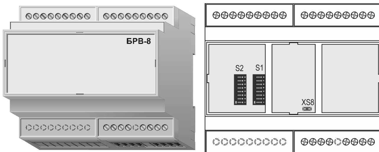
Рисунок 12 – Внешний вид блока, расположение переключателей.
