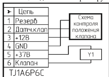
Рисунок 4 – Клапан КЗЭУГ.
