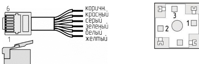
Вилка TP6P6C на кабель ЯБКЮ.685611.108-02
