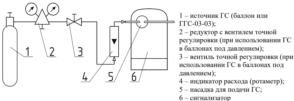
Рисунок Г.1 – Схема для настройки порогов срабатывания
