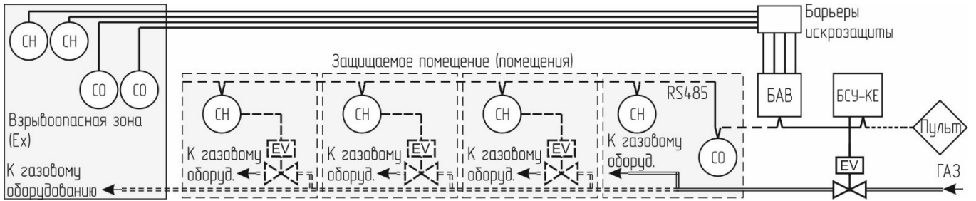
Рисунок 17 – Структура системы с интерфейсом RS485.
