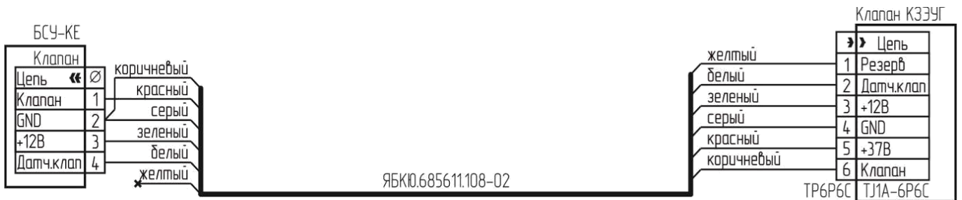
Рисунок А.2 – Типовая схема подключения клапана КЗЭУГ с разъемом TJ1A-6P6C
