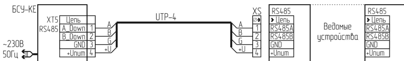
а) схема подключения сигнализаторов, пультов
