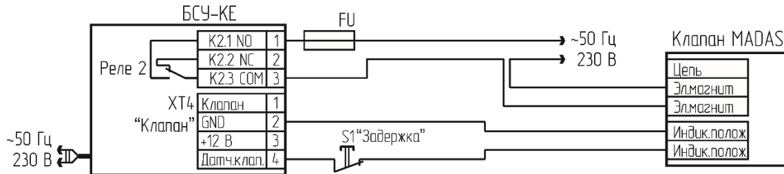
б) схема подключения клапана типа MADAS EVPS
