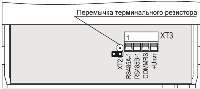
Рисунок Г.4 – Расположение разъемов ПД-Е(В)(Р)
