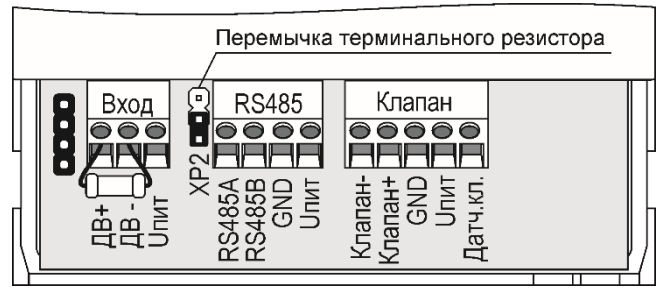
Рисунок Г.5 – Расположение разъемов СЗ-хЕ
