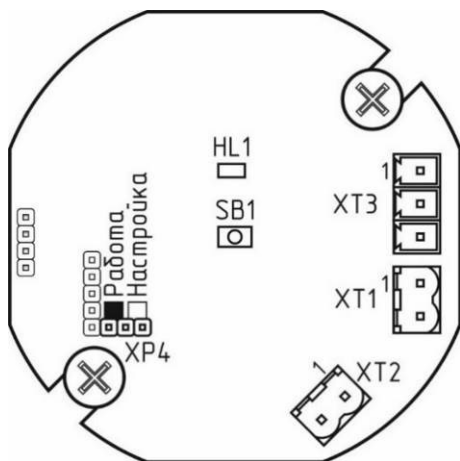
а) СЗ-1ДЛВ-420К/24
