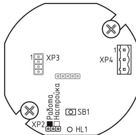
б) СЗ-2ДВ-420/24
