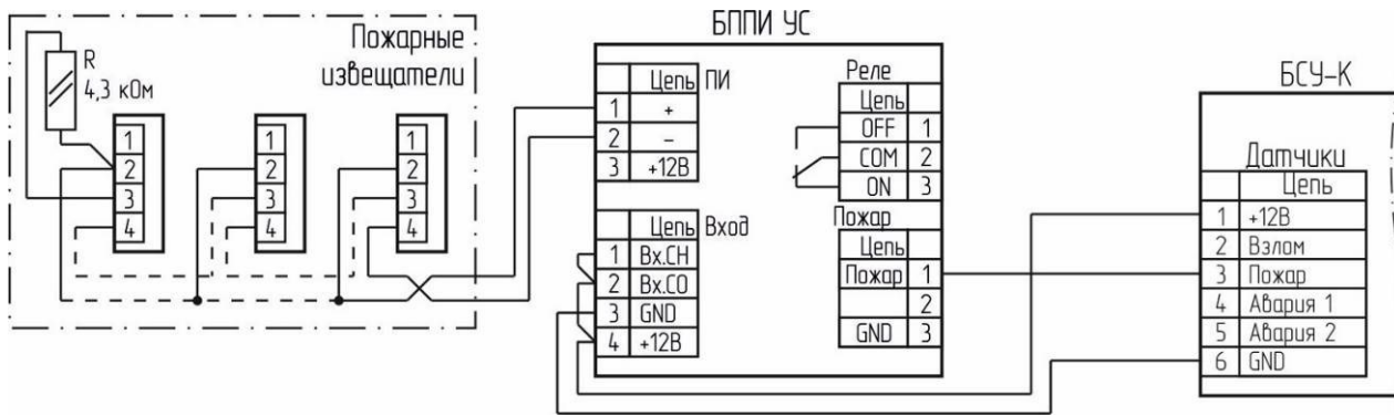
Рисунок В.10 – Схема подключения пожарных извещателей через блок БППИ УС.
