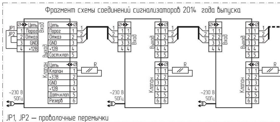
Рисунок В.1 – САКЗ-МК-3 с БСУ-К. Типовая электрическая схема соединений
