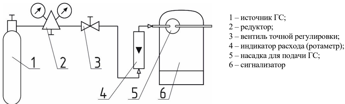
Рисунок Д.1 – Схема для настройки порогов срабатывания
