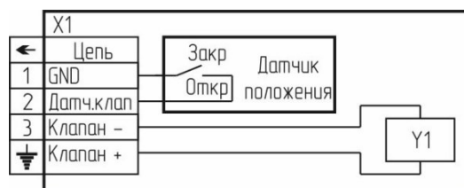
Рисунок 7 – Схема электрическая принципиальная.
