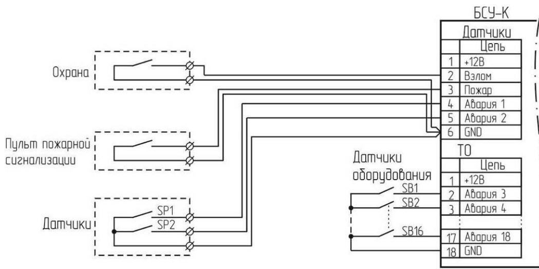
Рисунок В.8 – Нумерация разъемов кабелей.
