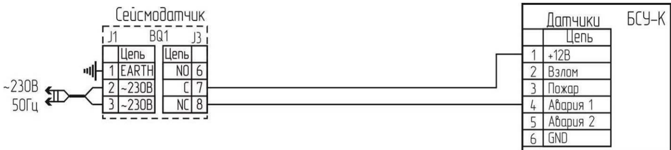
Рисунок В.5 – Типовая схема подключения сейсмодатчика
