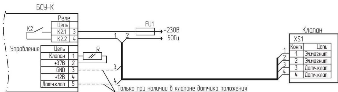
Рисунок В.2 – Типовая схема соединений для управления вентиляцией
