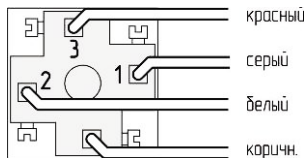
Розетка G2U3000-SK-1G на кабель ЯБКЮ.685611.109-01
