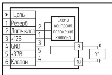
Рисунок 3 – Клапан КЗЭУГ. Схема электрическая принципиальная.
