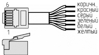
Вилка TR6P6C на кабель ЯБКЮ.685611.108
