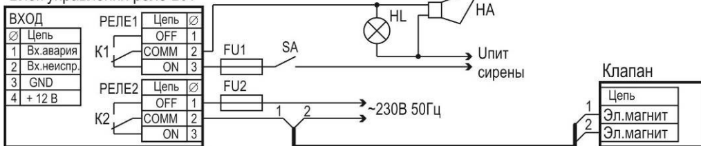
Рисунок 1 – Блок управления реле БУР. Типовая схема подключения.
