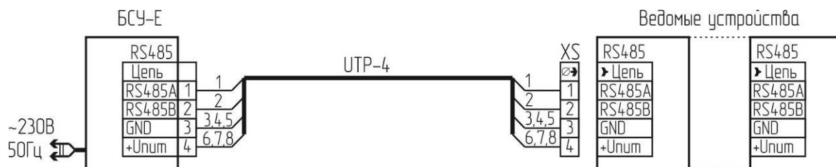
Рисунок 6 – Схема соединений для программирования адресов
