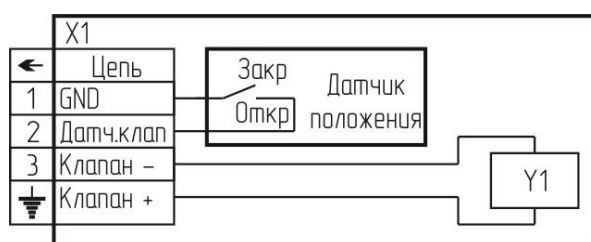
Рисунок 5 – Клапан КЗГЭМ-У. Схема электрическая принципиальная.
