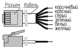
Вилка на кабель TP6P6C (цвета проводов)
