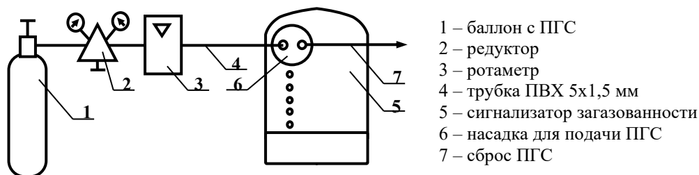
Рисунок Е.1 – Рекомендуемая схема подачи ГС на сигнализатор
