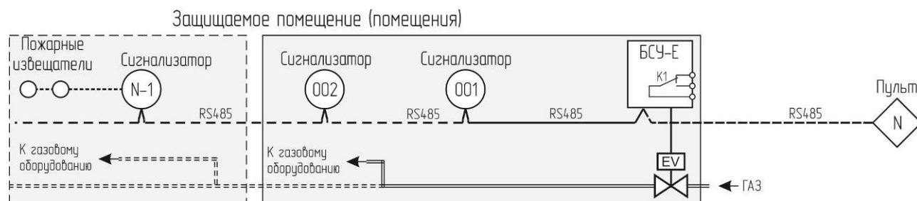
Рисунок 7 – Структура системы с RS485 и групповой защитой.
