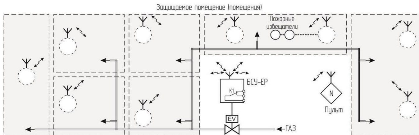
Рисунок 11 – Структура системы с радиоканалом и групповой защитой.
