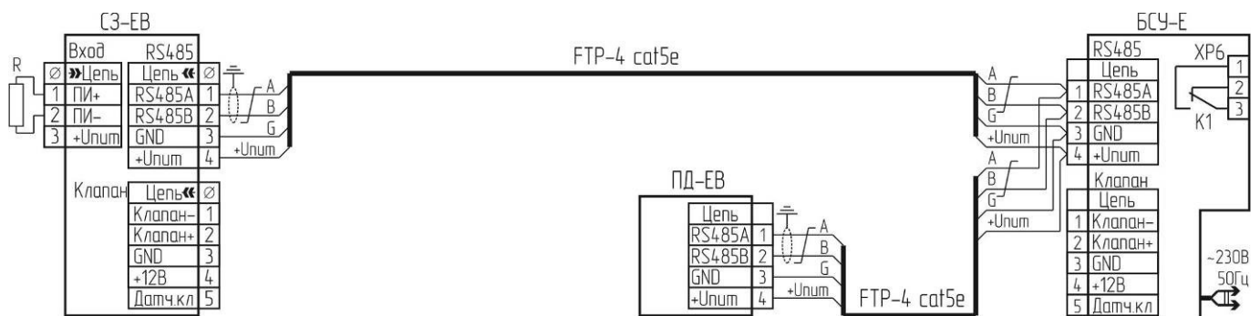
Рисунок В.3 – Нумерация разъемов кабелей.
