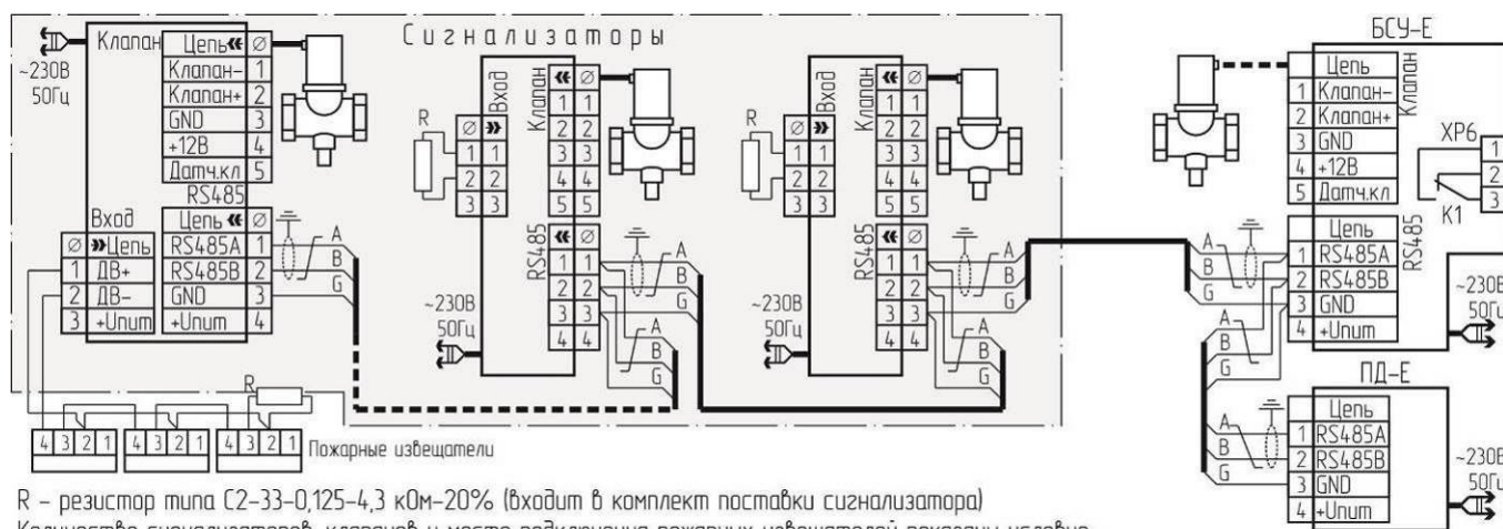
Рисунок 10 – Схема соединений системы с RS485 и индивидуальной защитой.
