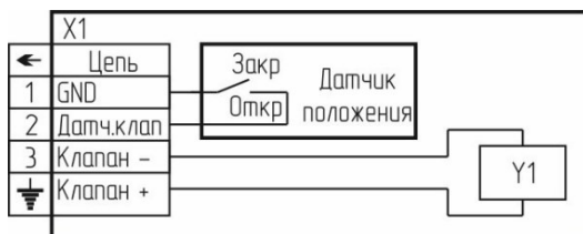
Рисунок 5 – Клапан КЗГЭМ-У.
