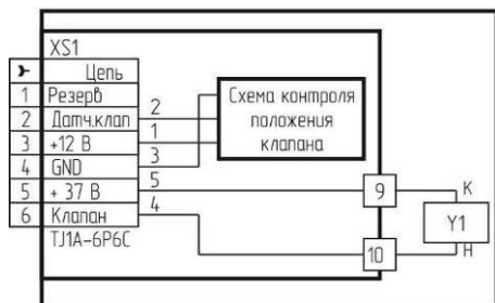
Рисунок 3 – Клапан КЗЭУГ.
