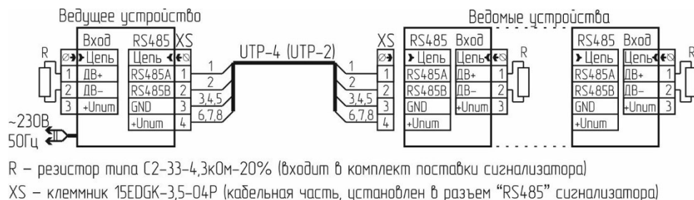
Рисунок 7 – Схема для программирования адресов
