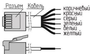
Вилка на кабель TP6P6C (цвета проводов)
