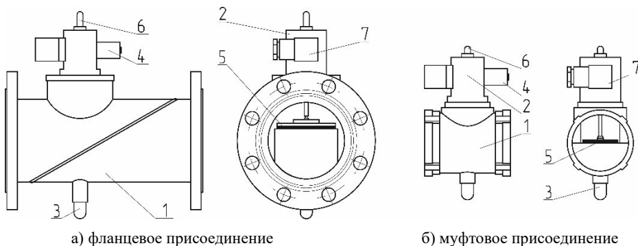
Рисунок 4 – Внешний вид клапана КЗГЭМ-У
