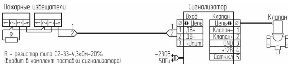
Рисунок 9 – Схема соединений с одним сигнализатором без пульта.
