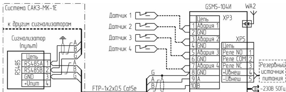
Рисунок В.4 – Схема подключения извещателя GSM5-104И.
