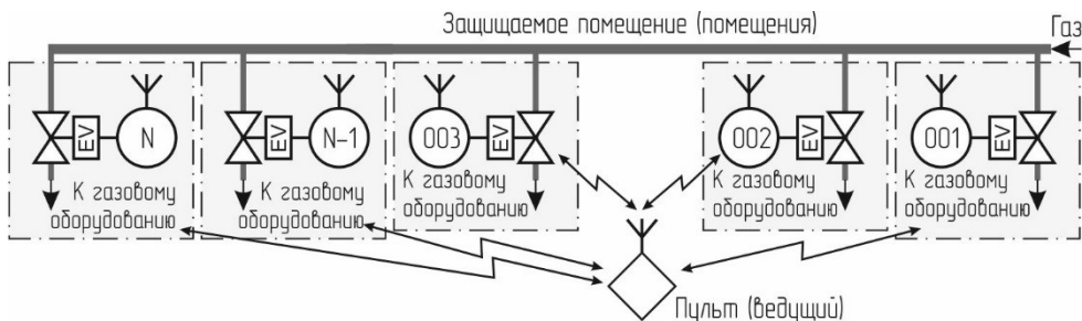
Рисунок 21 – Система с индивидуальной защитой и связью по радиоканалу
