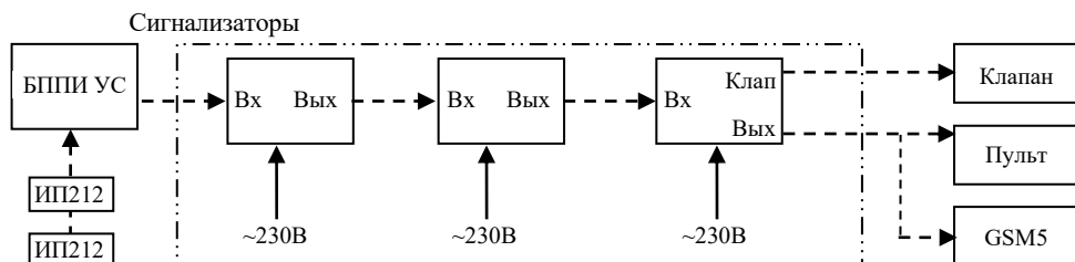
Рисунок 1 – Структурная схема
