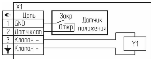
Рисунок 6 – Клапан КЗГЭМ-У.
