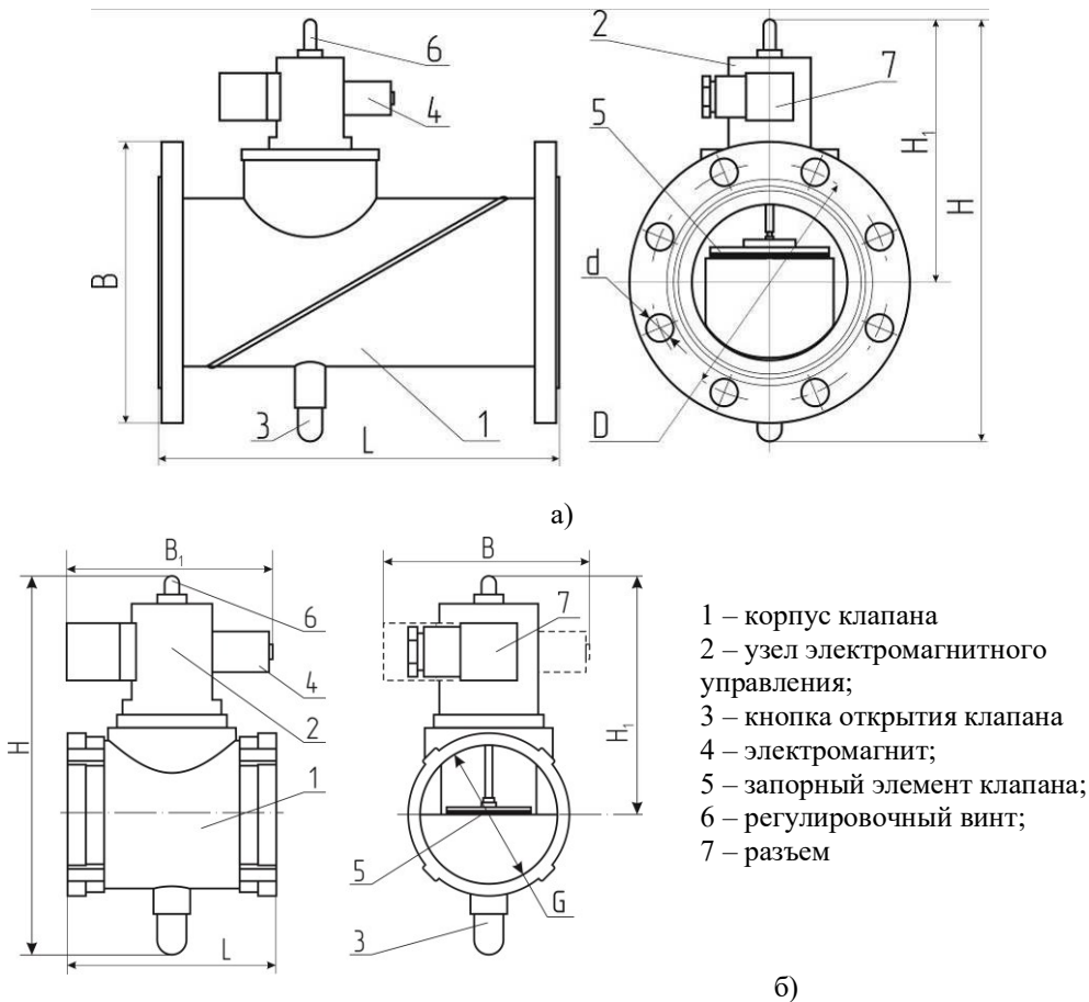
Рисунок 2 – Внешний вид клапана: а) фланцевый; б) муфтовый
