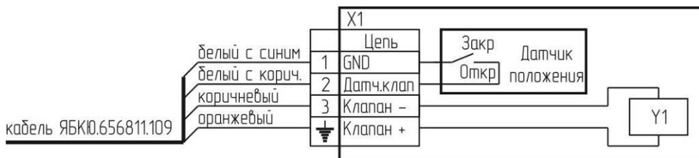
Рисунок 1 – Схема электрическая принципиальная клапана
